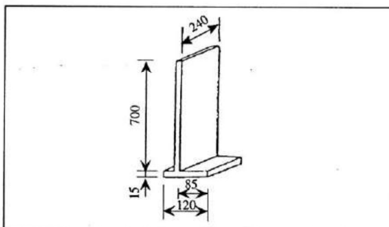
Figure 2 : Elément du mur.
