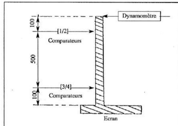
Figure 3 : Dispositif de mesures
