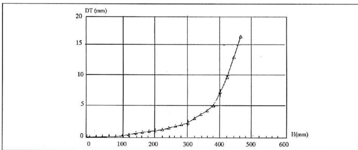
Figure 5 : Courbe de référence du sable seul. DT = f(H) .
